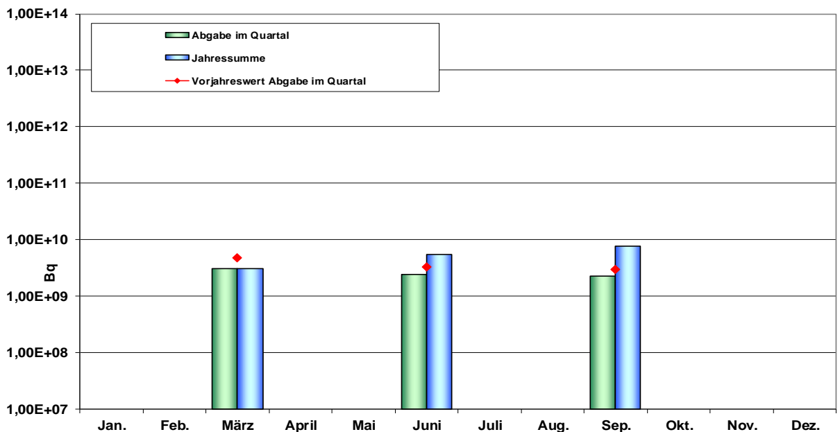
Abgabe radioaktive Gase mit der Kaminfortluft 2024
